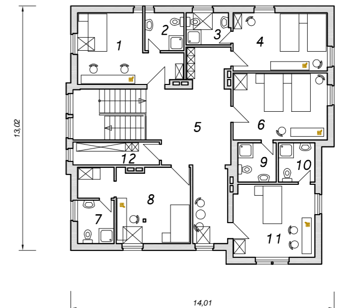
DACHGESCHOSS 142,05 m 2
